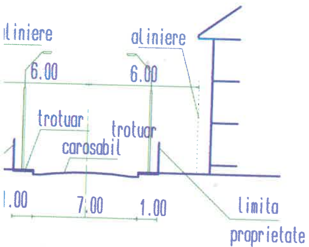
PROFIL STRADAL A-A
